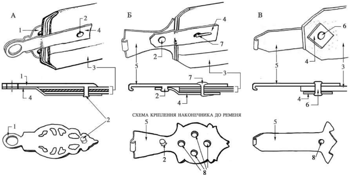
Рис. 3. Способи фіксації металевих наконечників до плоских ремнів накидної частини застібки: а – з'єднання паянням та клепаанням литників; б – з'єднання клепаанням литників та цвяхами; в – з'єднання на клепки. 1 – петля на пластині, 2 – літник, 3 – плоский ремінь, 4 – фіксуюча пластина, 5 – гачок, 6 – заклепка, 7 – зігнутий цвях, 8 – наскрізні отвори для цвяхів, заклепок та елементи оздоблення
