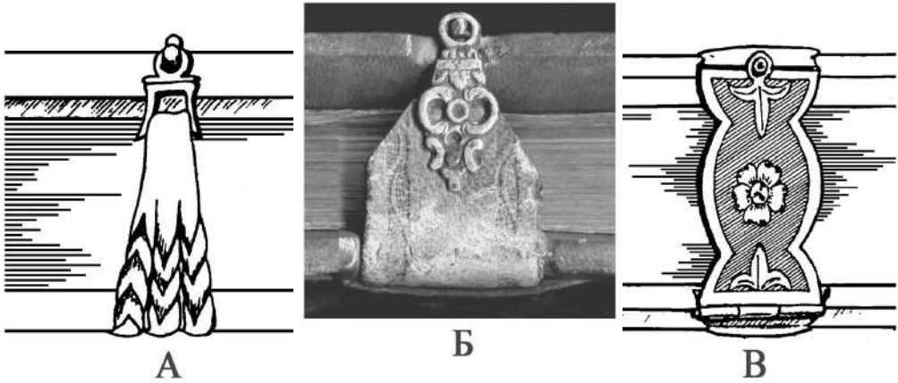
Рис. 2. Типи шпенькових застібок: а – класична візантійська застібка на тричастинному ремні; б – застібка на накладний шпеньок; в – застібка на вертлюзі
